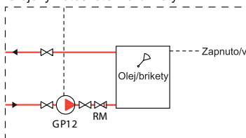
Olejový kotel/kotel na brikety
