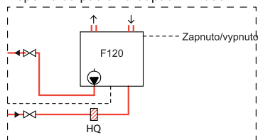
Tepelné čerpadlo na odpadní vzduch
