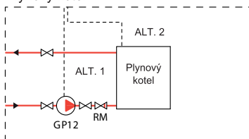
Plynový kotel
